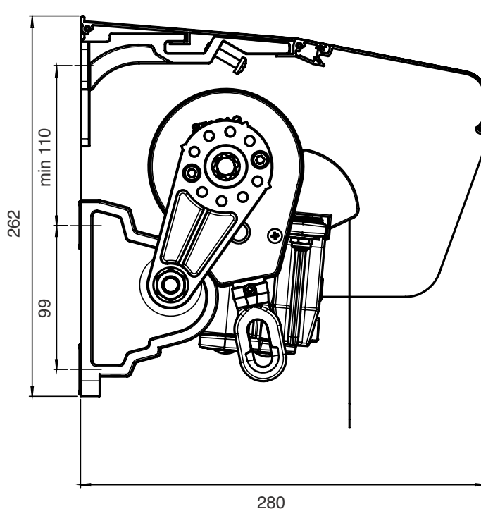
Montáž na stěnu s převodovkou a střechou
