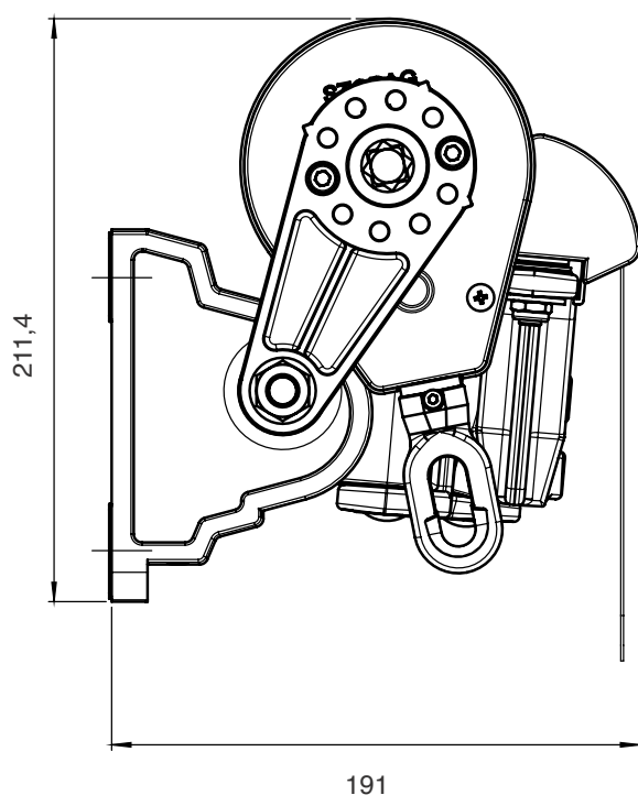
Montáž na stěnu s převodovkou
